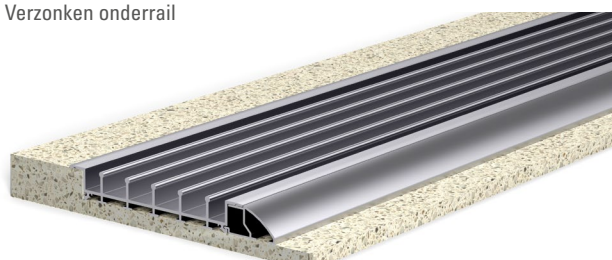
Verzonken onderrail met zijprofiel
